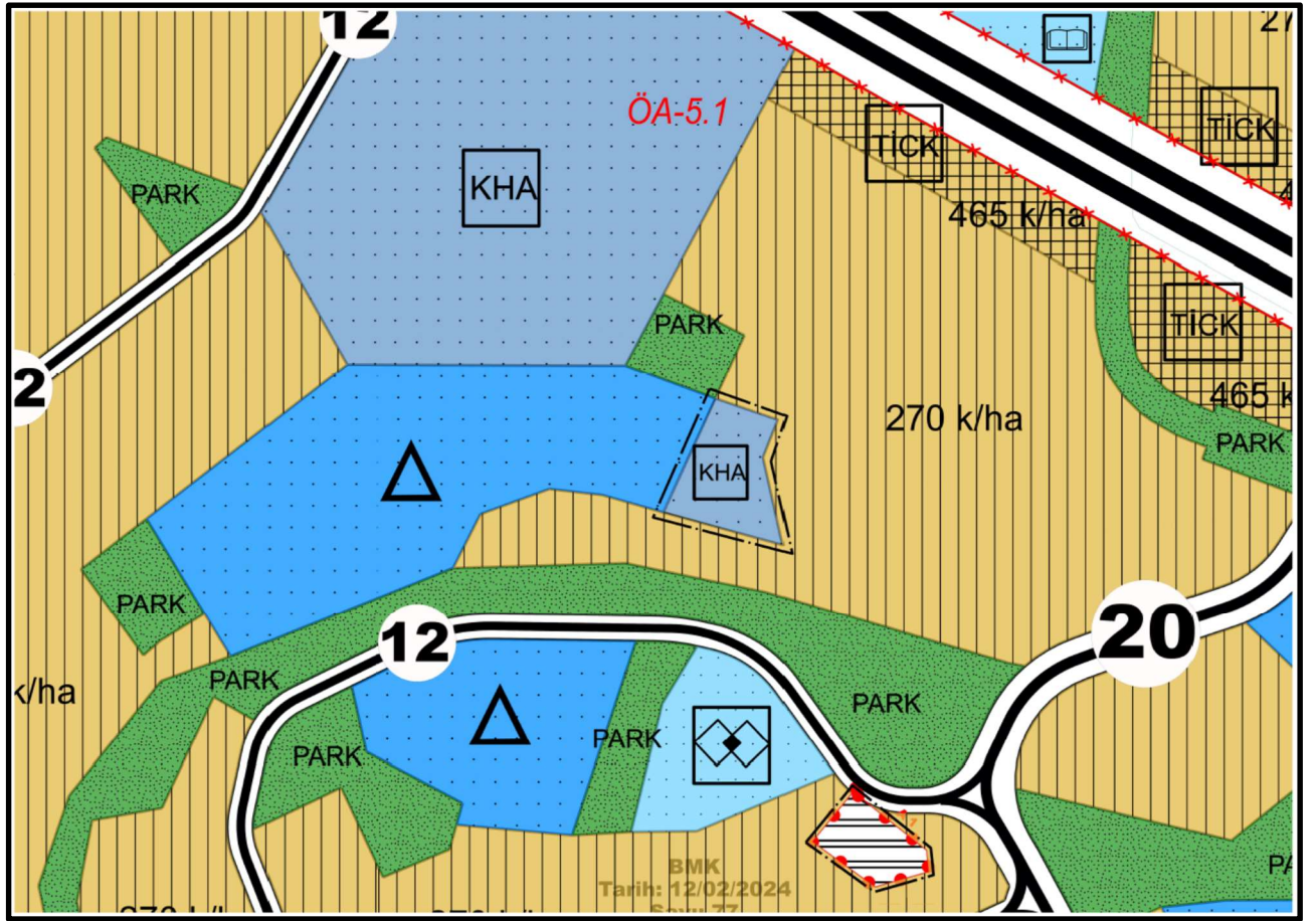
Harita 3: Onaylı 1/5000 Ölçekli Nazım İmar Planı Değişikliği
