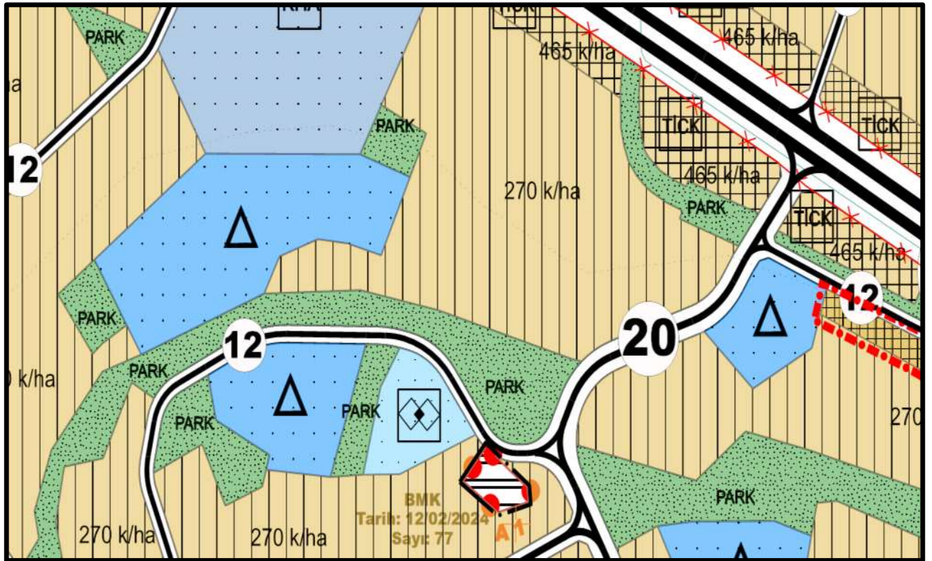
Harita 2: Onaylı 1/5000 Ölçekli Nazım İmar Planı
