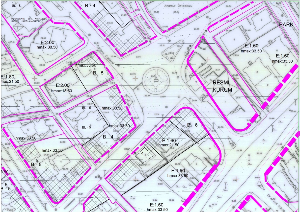
Şekil 2. 1/1000 ölçekli Uygulama İmar Planı
