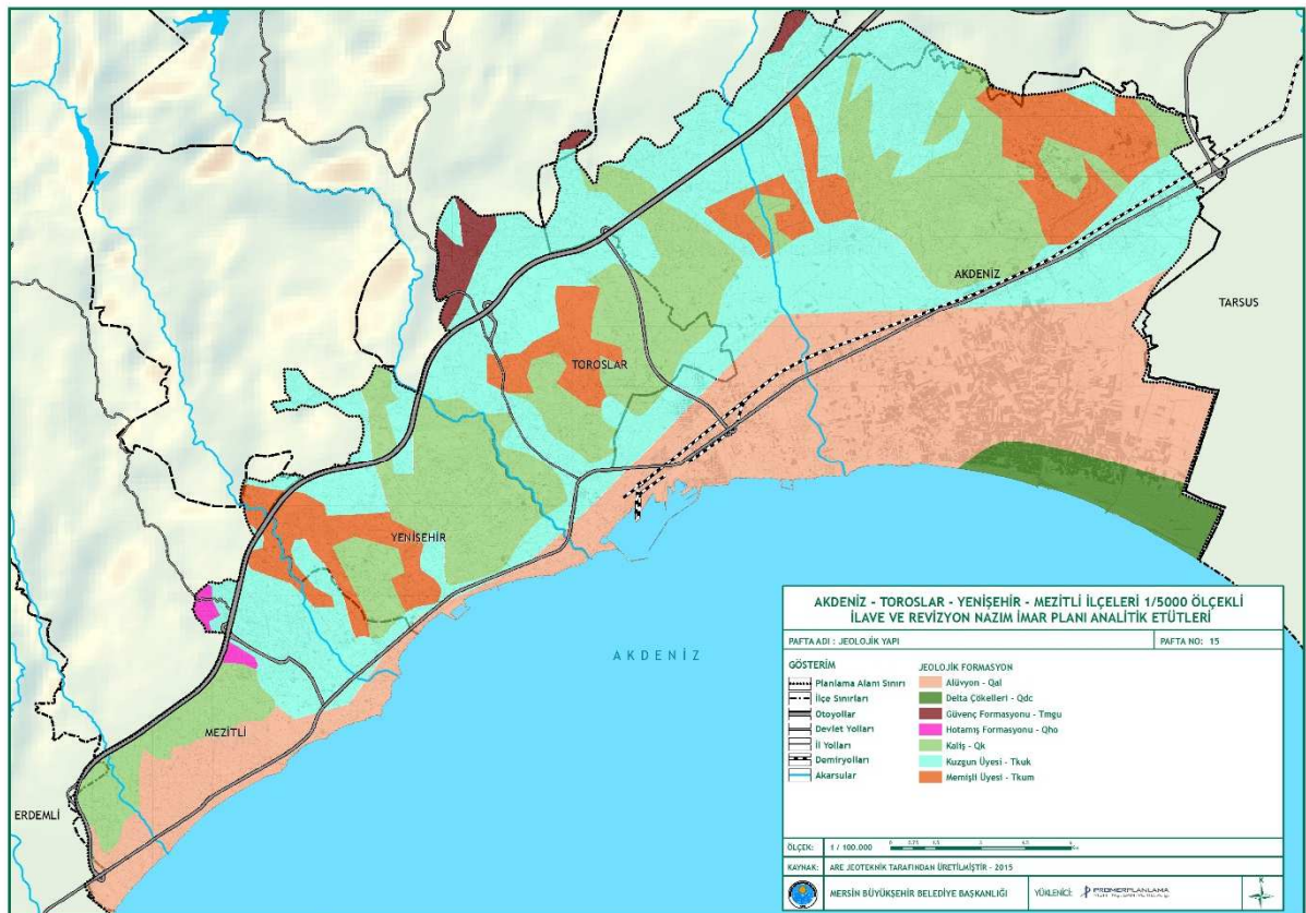
Şekil 11. Jeolojik Formasyon
