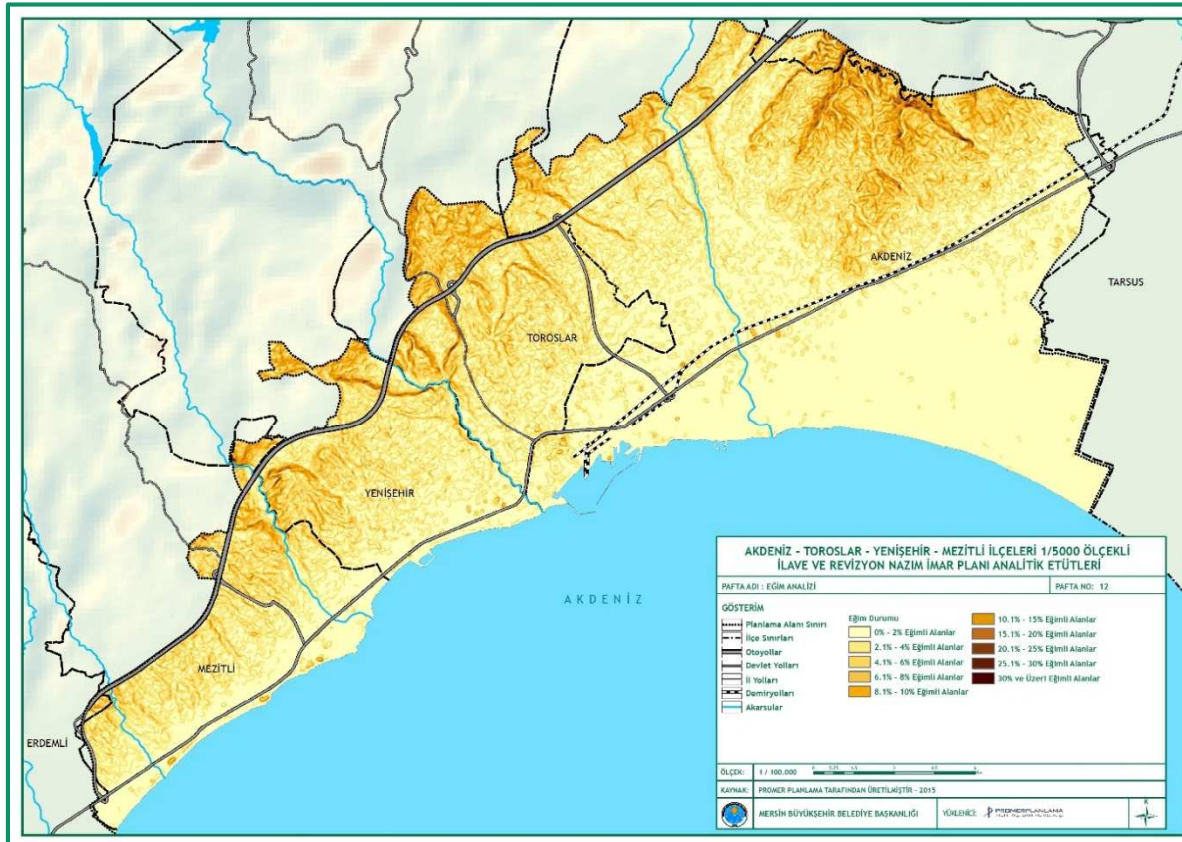
Şekil 10. Eğim Durumu
