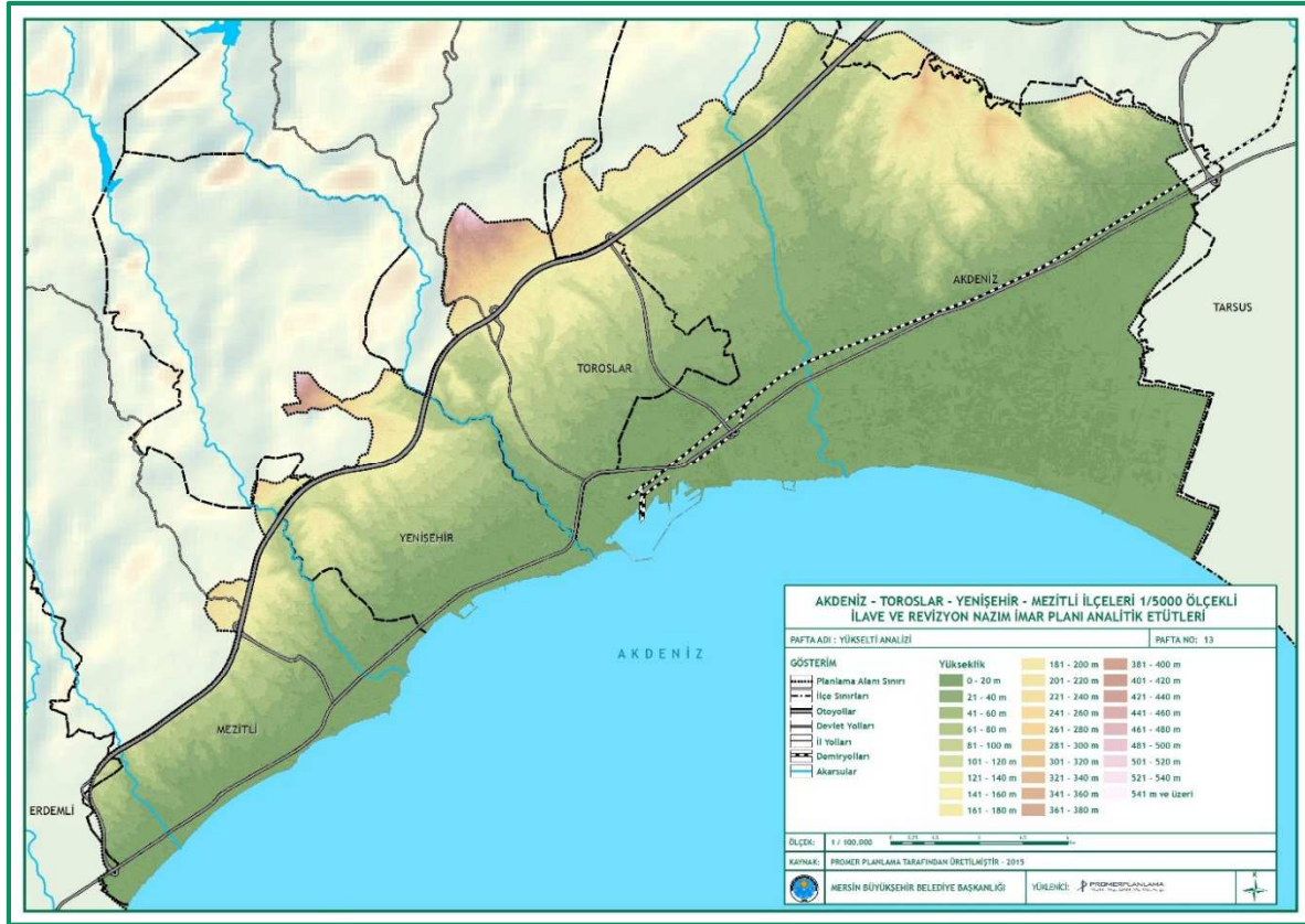
Şekil 9. Yükselti Kuşakları
